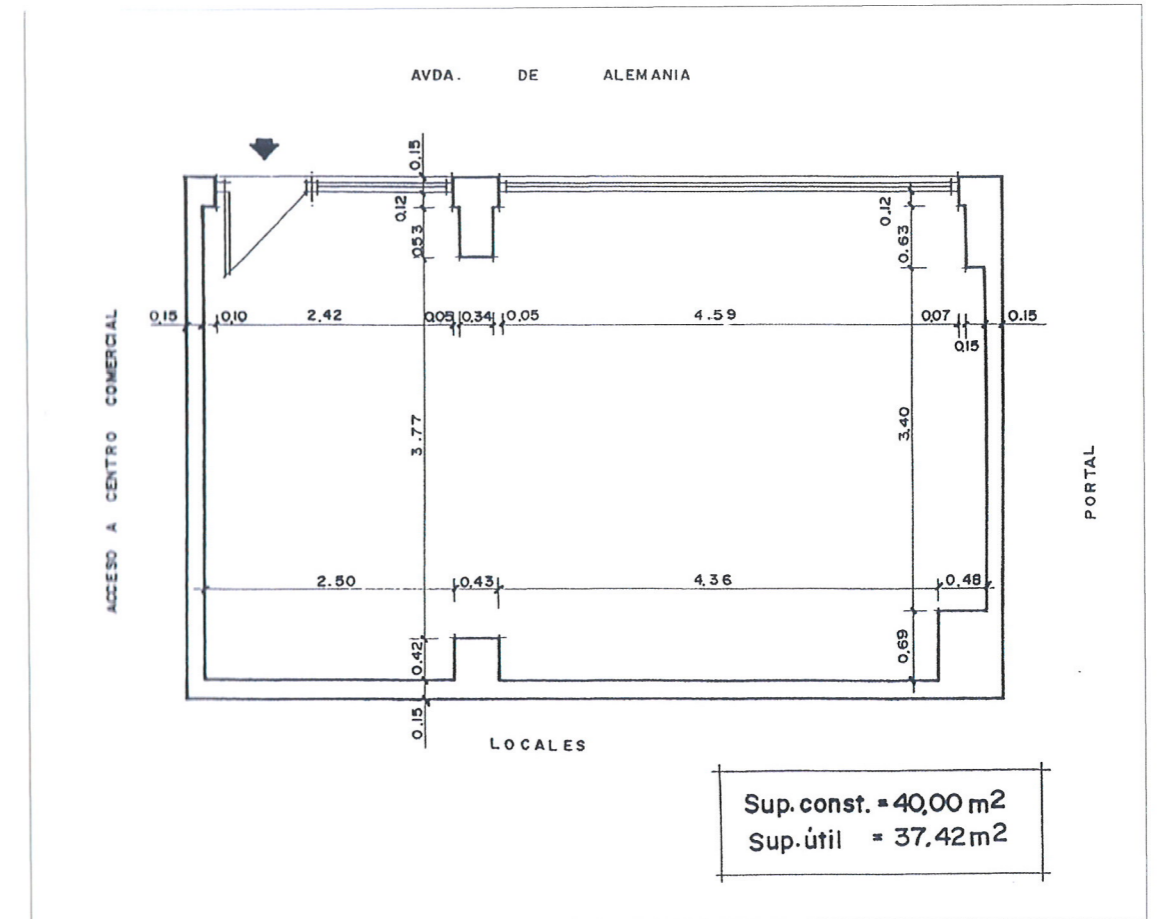
PLANTA
