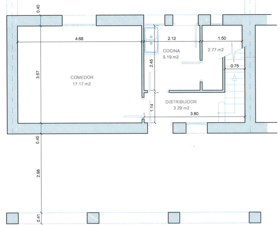
PLANTA BAJA Nº 3
