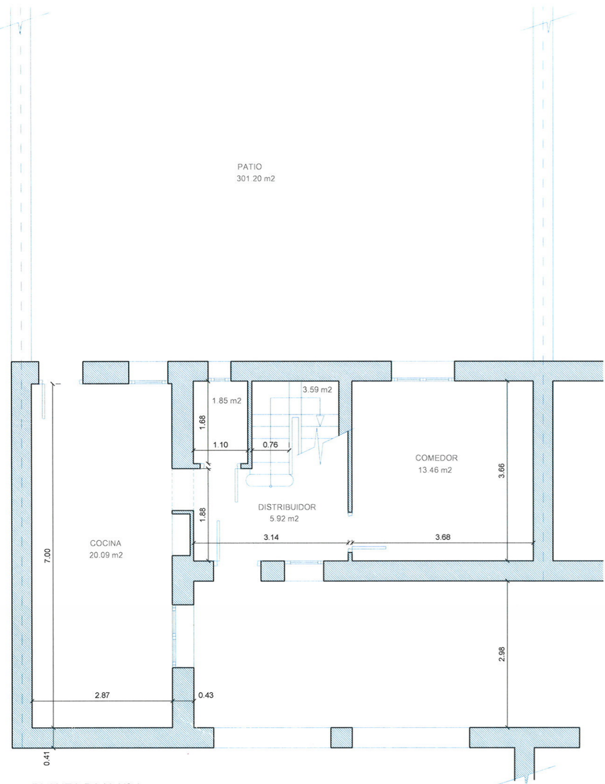
PLANTA BAJA Nº 4
