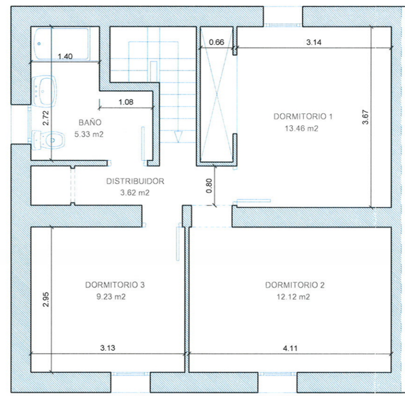
PLANTA PRIMERA Nº 4
