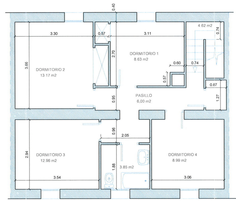
PLANTA PRIMERA Nº 3
